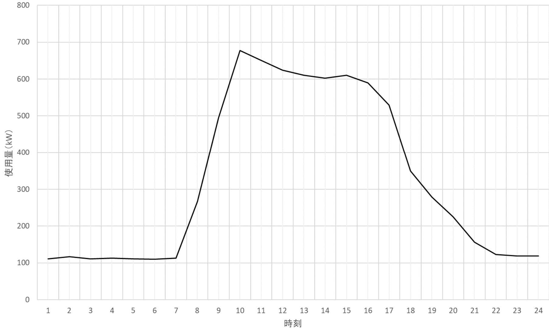
予定最大負荷日のロードカーブ
